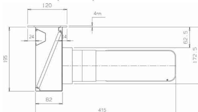
URS Vooraanzicht (omkeerbaar)
