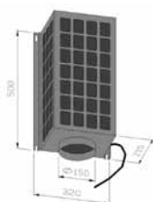
Airodesign by O+F A-Line Plasmarecirculatiefilter met 3 elektroden
