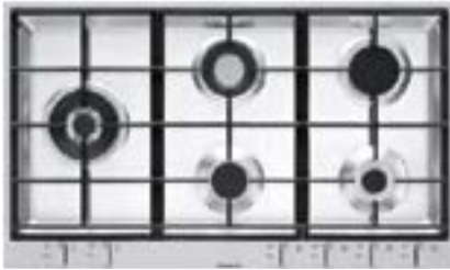
90 cm B_Free opbouw kookplaat 3 gas branders + dubbele ring Chef + dubbele ring 4 kW
