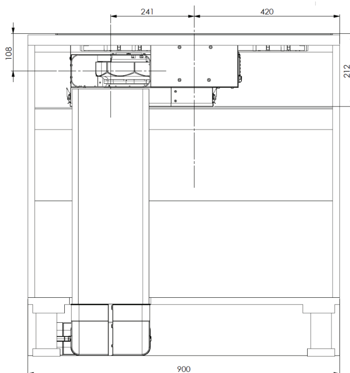
Achteraanzicht van een 90 cm brede kast
